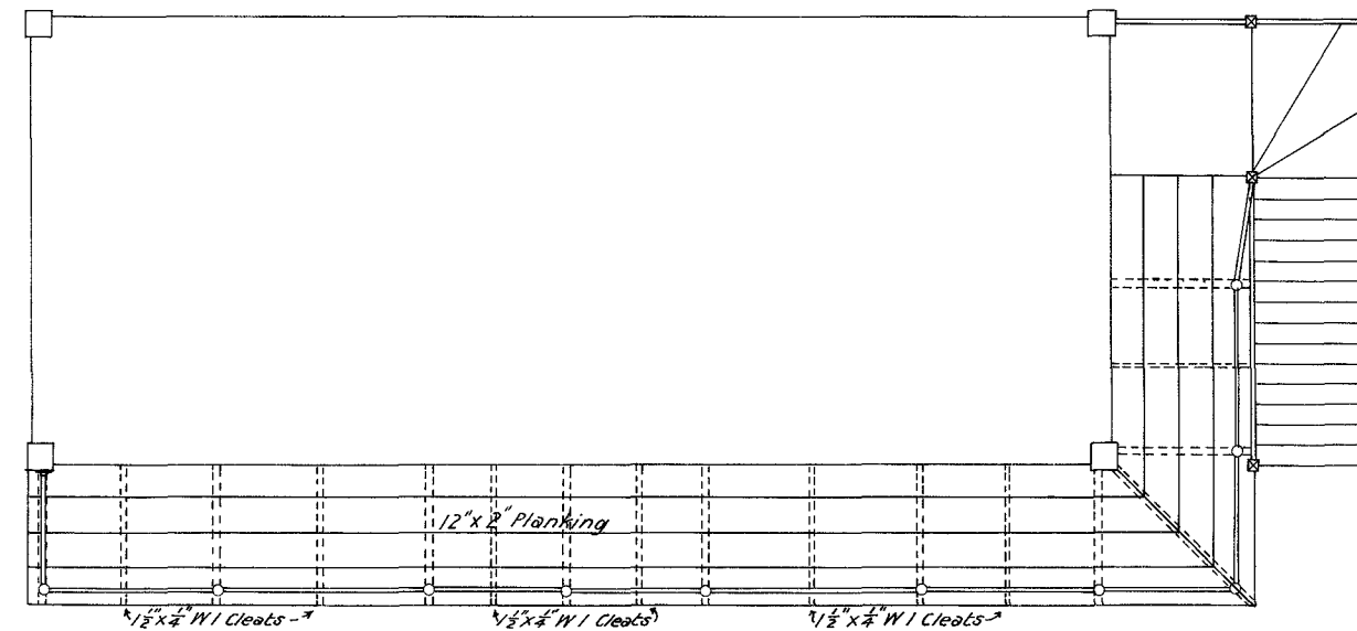
— Plan —
