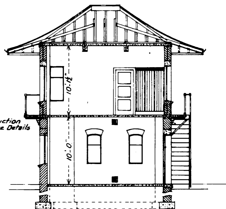
LONGITUDINAL SECTION
