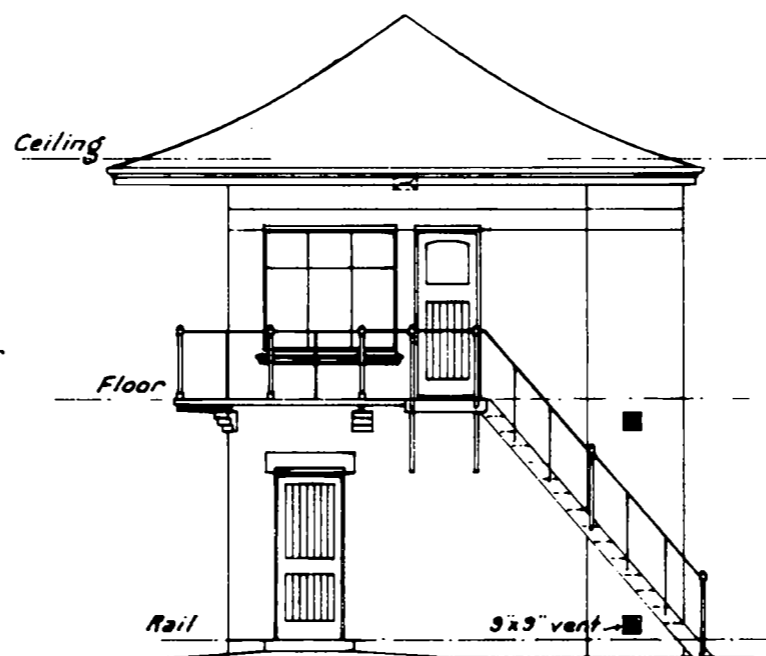
END ELEVATION
